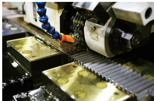
ラックギヤの歯切り工程
