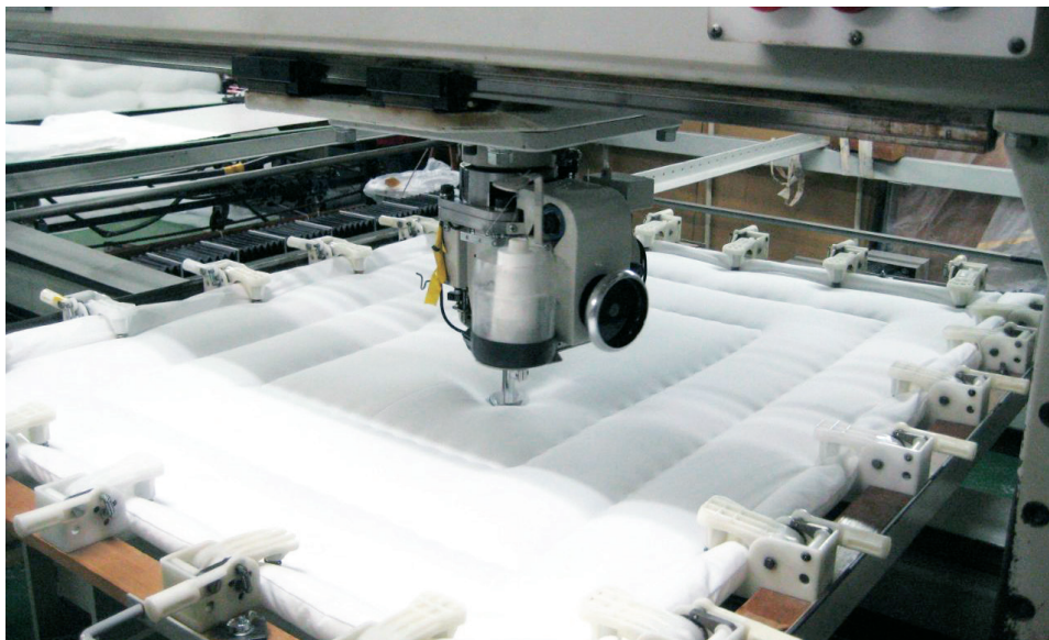
自動キルティングマシン
